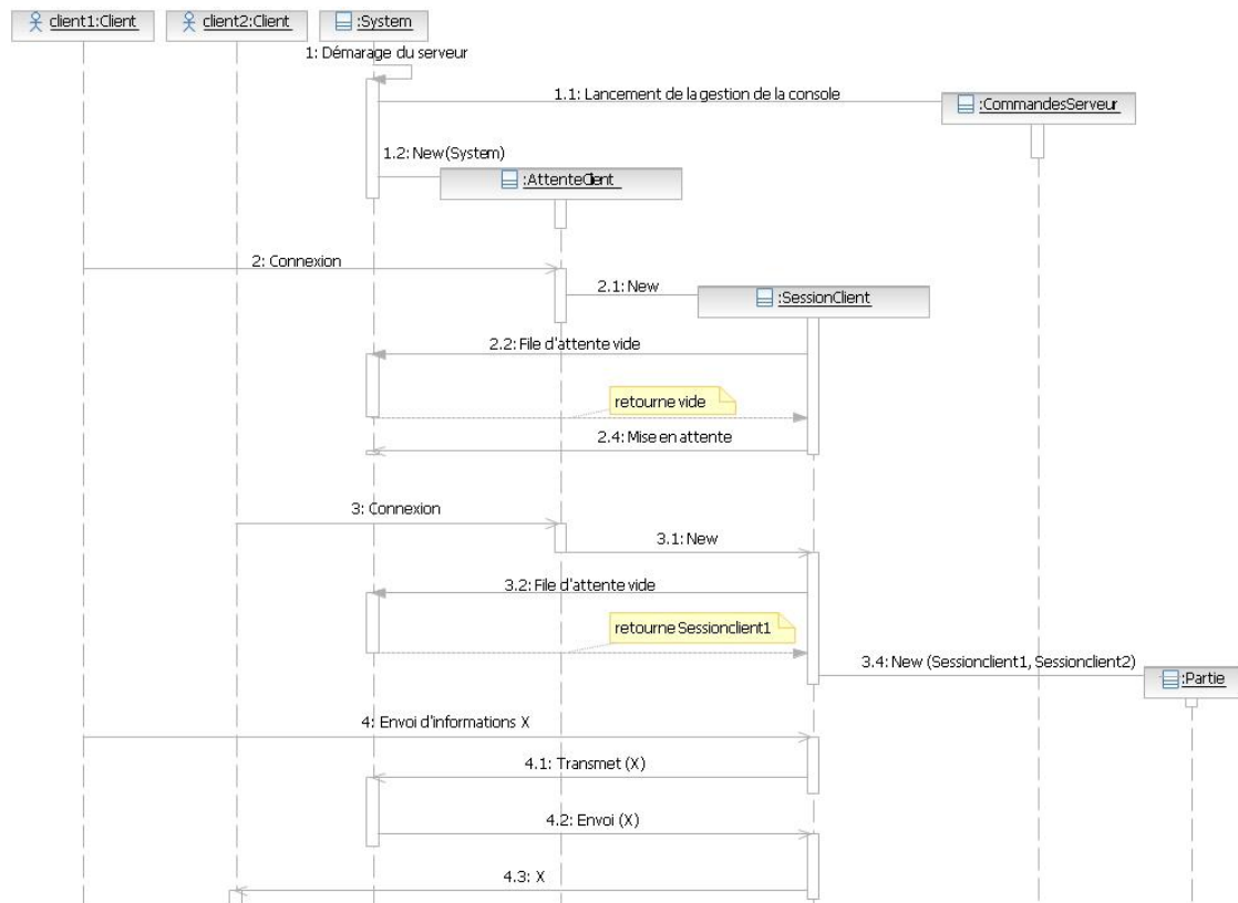
Figure 10 Interaction séquentielle client-serveur
